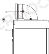
CONDOTTO COASSIALE Ø 60-100
