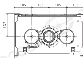
VISTA DALL'ALTO
