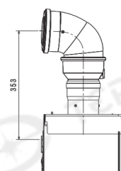
CONDOTTO COASSIALE Ø 80-125
